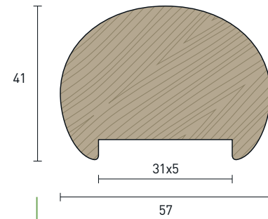
Corrimano arrotondato scanalato
