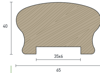
Corrimano sagomato scanalato
