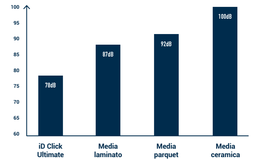
Rumore al calpestio all'interno della stanza (dB)
