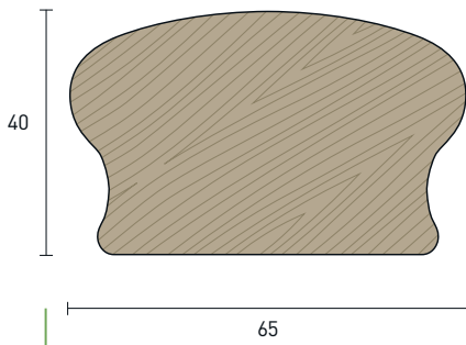
Corrimano sagomato
